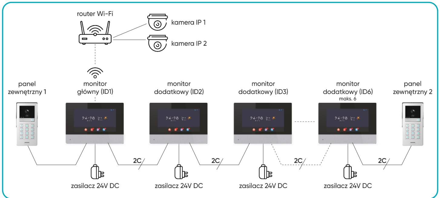
rys. 7 Schemat podłączenia zestawu jednorodzinnego.
