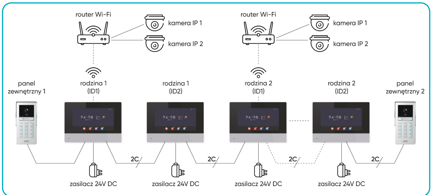
rys. 8 Schemat podłączenia zestawu dwurodzinnego.
