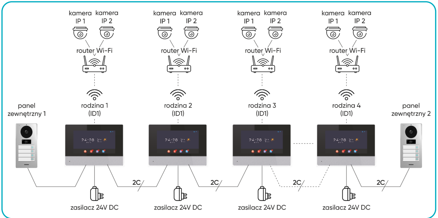
rys. 9 Schemat podłączenia zestawu czterorodzinnego.
